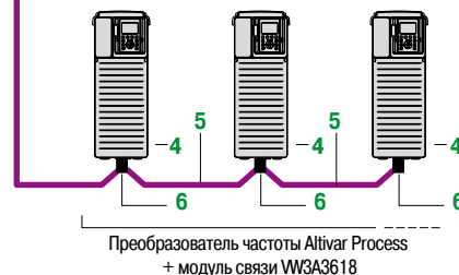
Шина CANopen (3)
