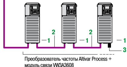
Шина CANopen (3)
