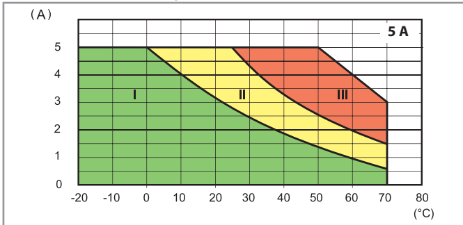
L77-1 Зависимость тока выход. цепи от температуры 77.01.9.024.805x при 32 В DC
